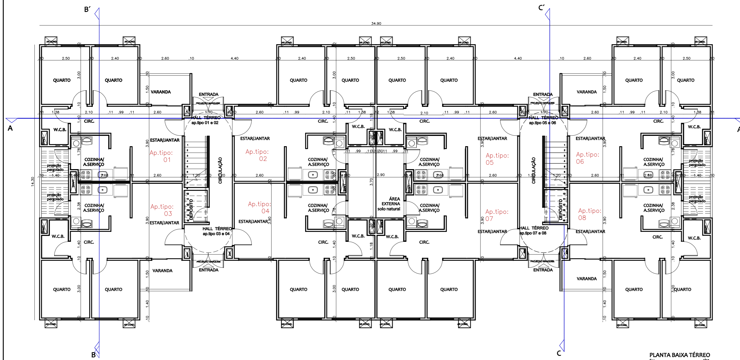
PLANTA BAIXA TÉRREO Esc. 1/50
