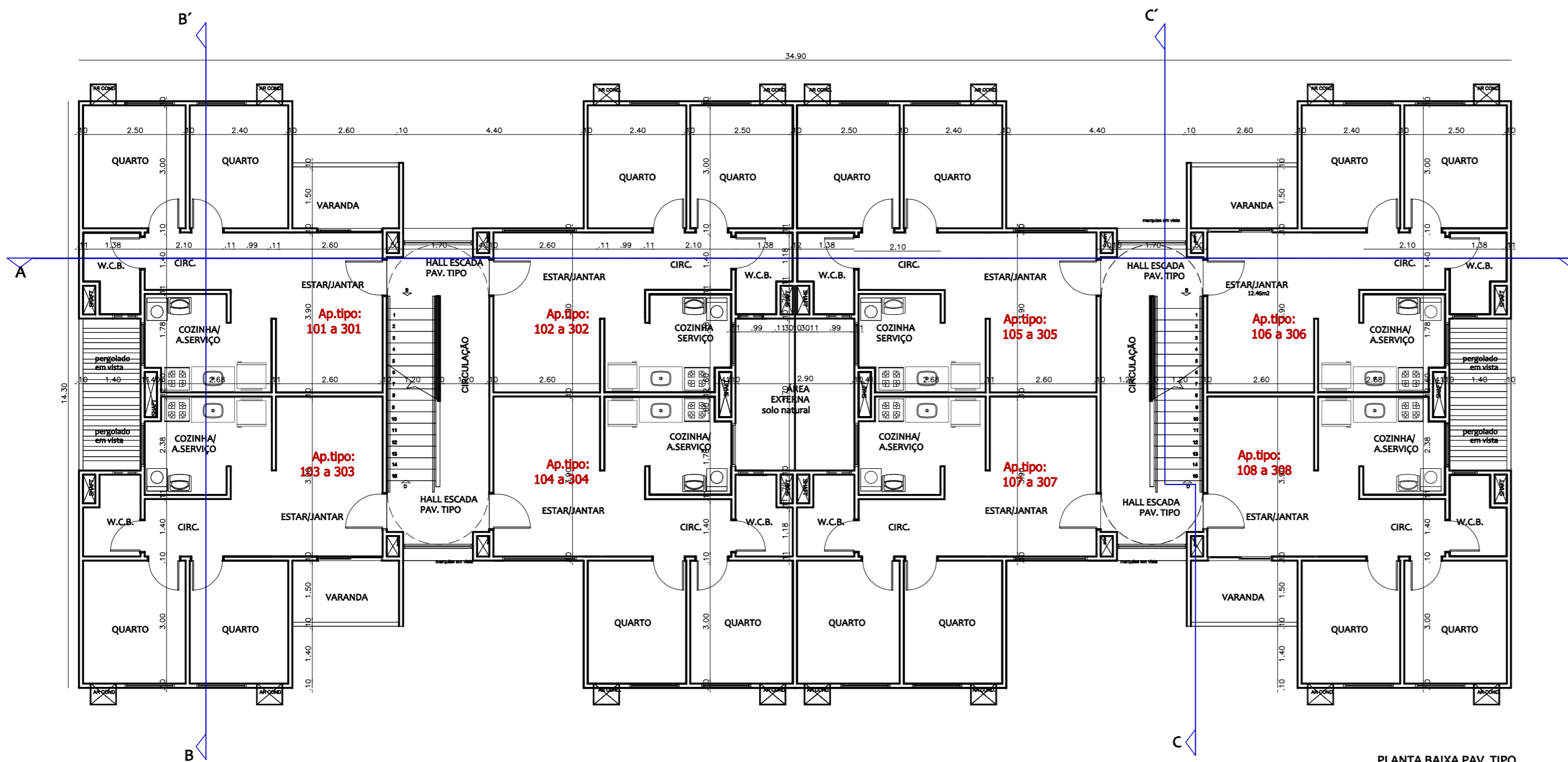
PLANTA BAIXA PAV. TIPO Esc. 1/50
