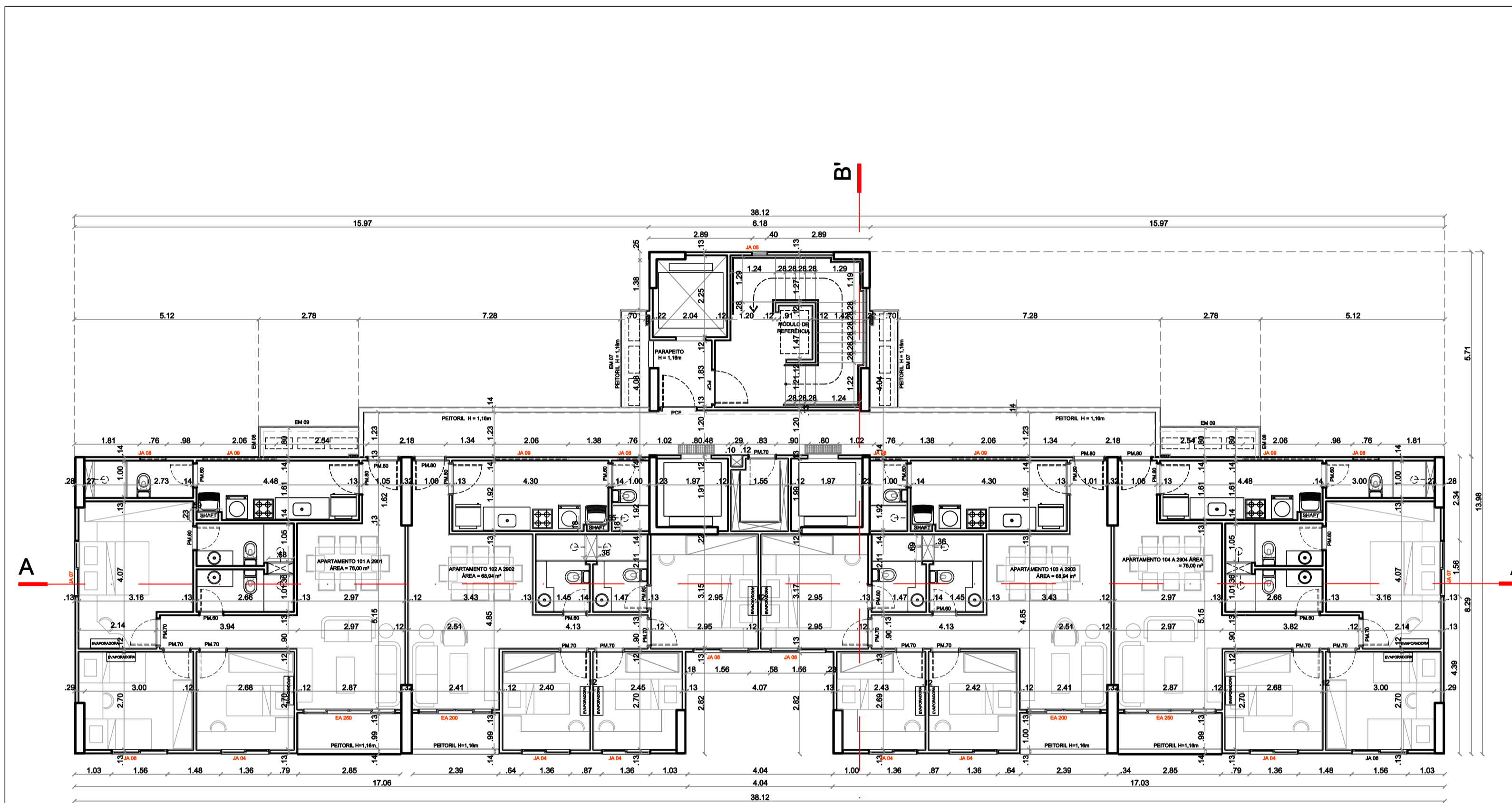
PLANTA BAIXA - PAVIMENTO TIPO ESCALA 1/100
