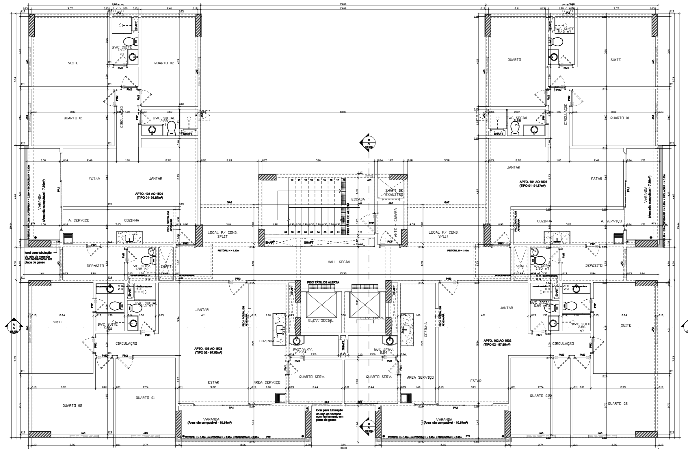
PLANTA BAIXA - PAV. TIPO ESCALA 1/100
