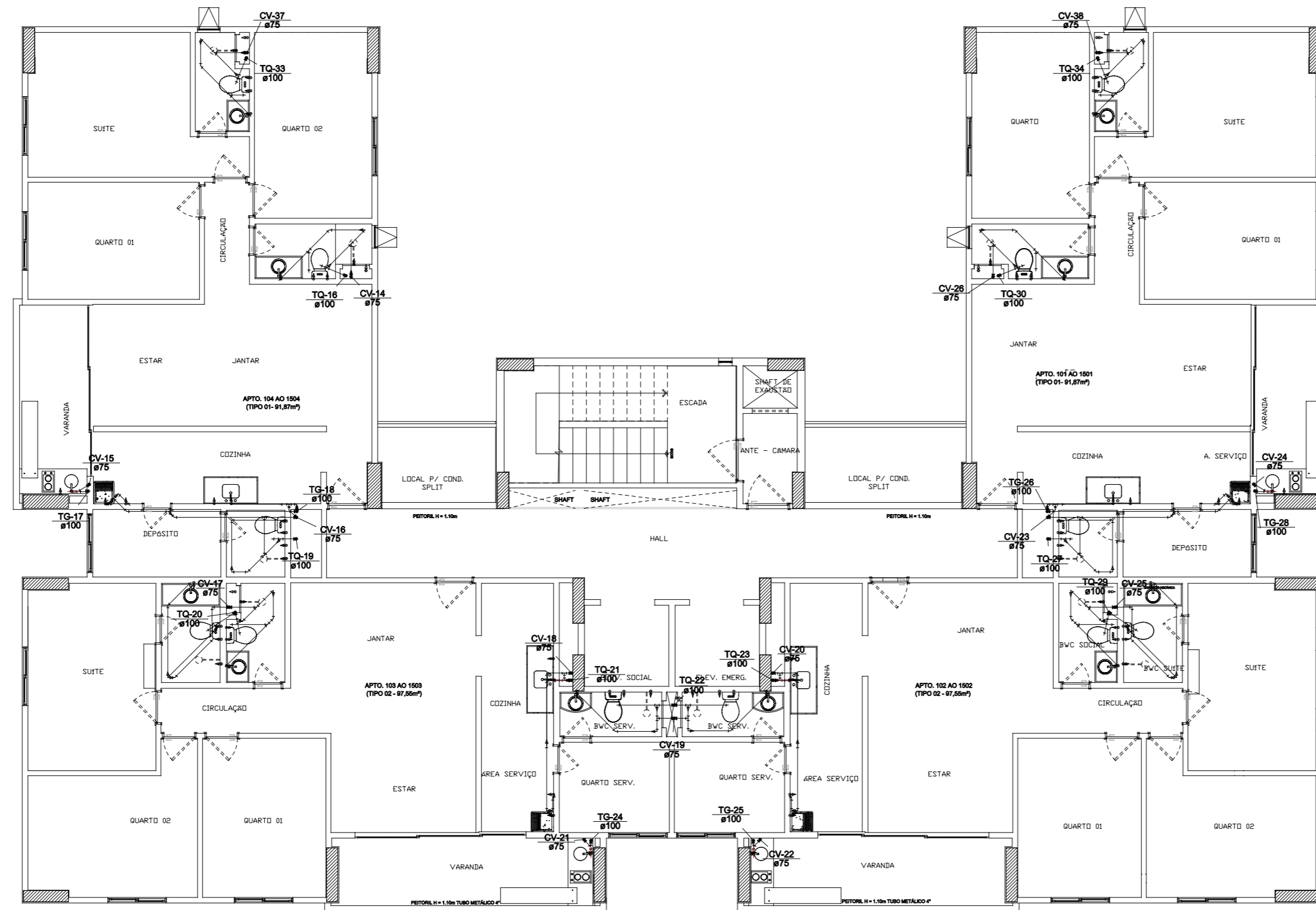
PLANTA BAIXA DE HIDRÁULICA - PAV. TIPO ESCALA _____ 1/100
